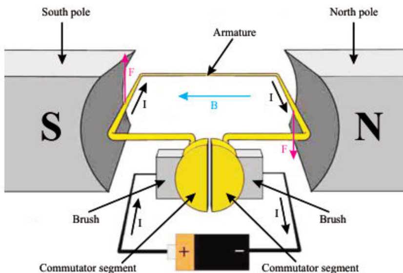
Fig: 16.11. Turning effect on D.C motor
