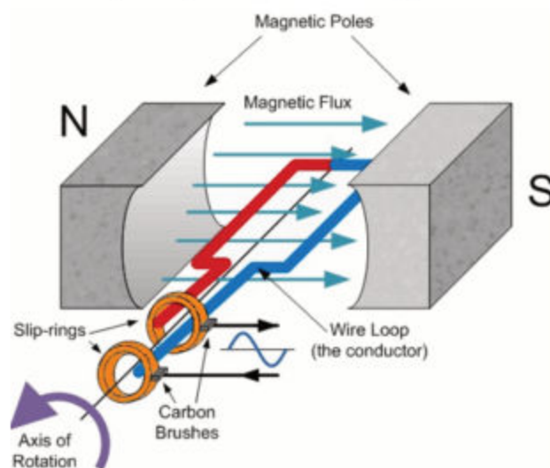
Fig: 16.16 A.C generator
