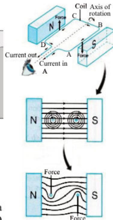
Fig: 16.12 Torque on D.C motor
